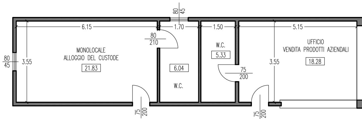
B-Superfetzung interna della serra pianta sc. 1:100
