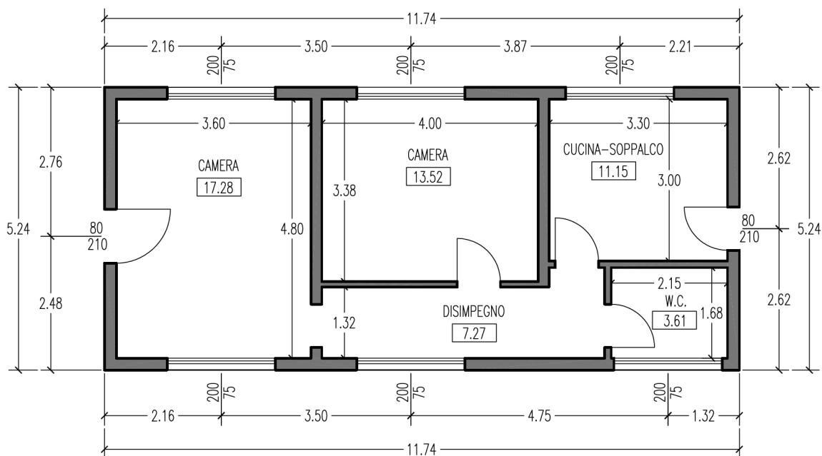
F-deposito (attualmente a uso residenziale) pianta sc. 1:100
