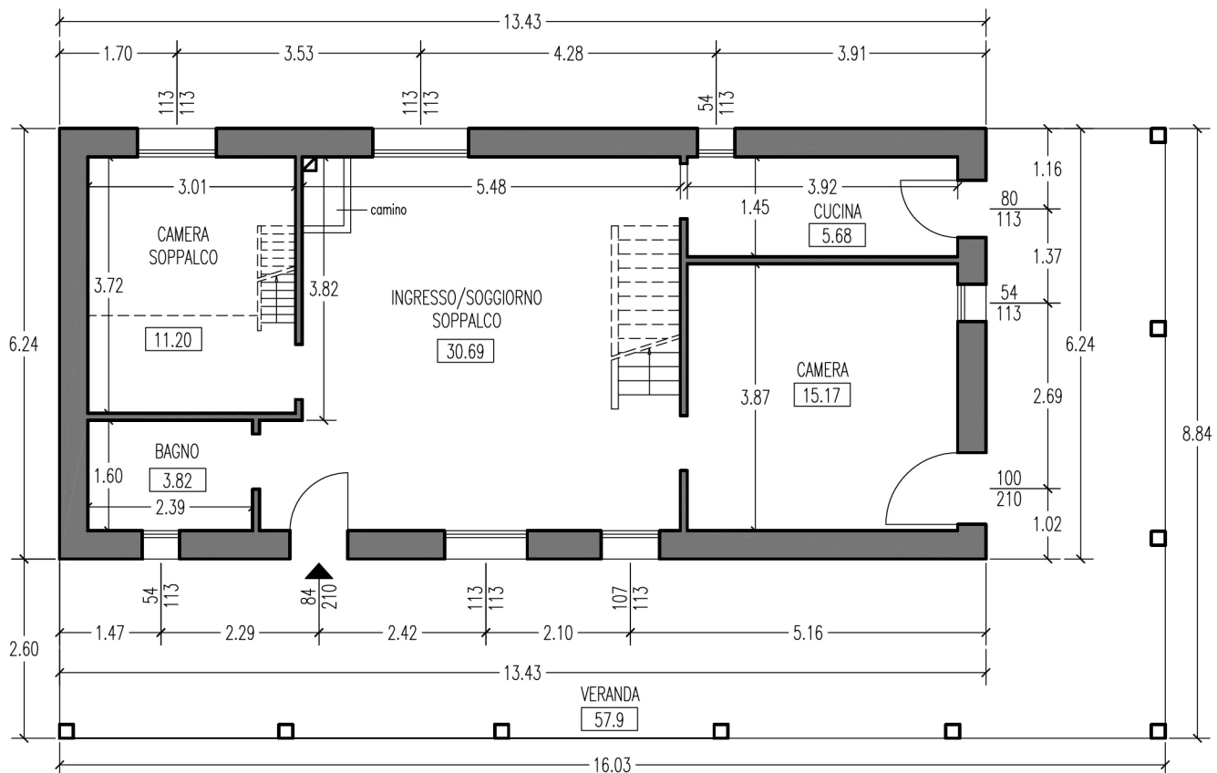
D-alloggio del custode del fondo pianta sc. 1:100
