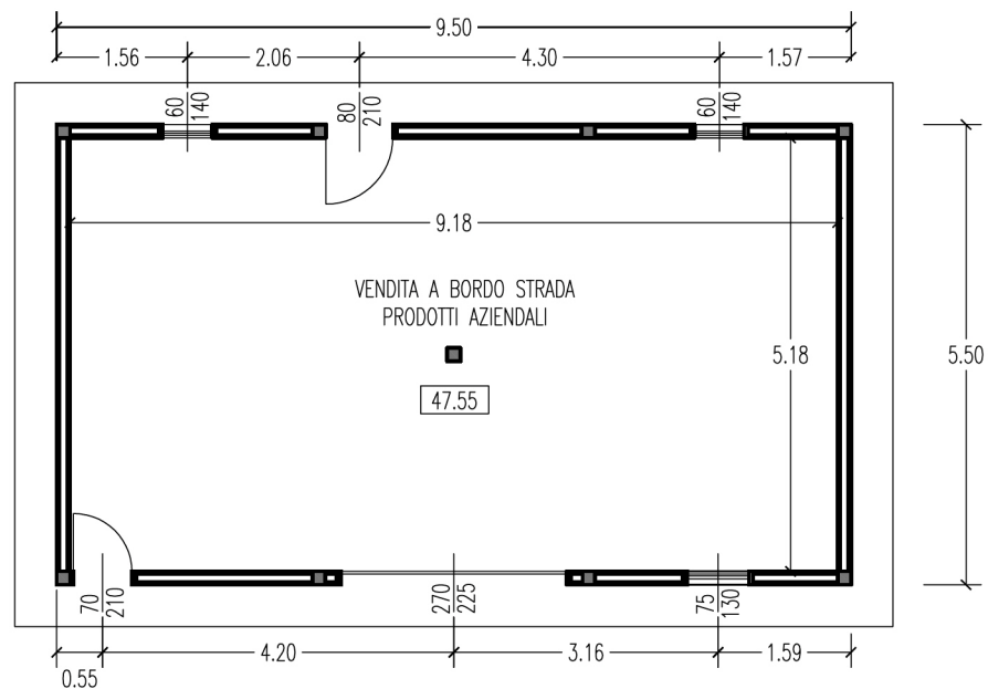
C-vendita a bordo strada prodotti aziendali pianta sc. 1:100
