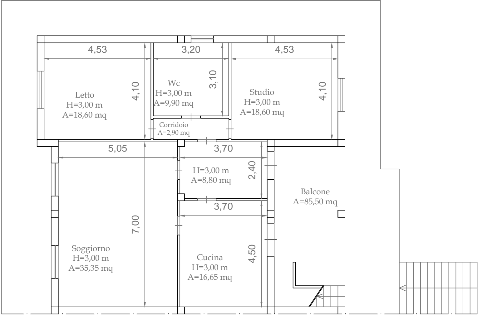
Pianta Piano Primo - Scala 1:100
