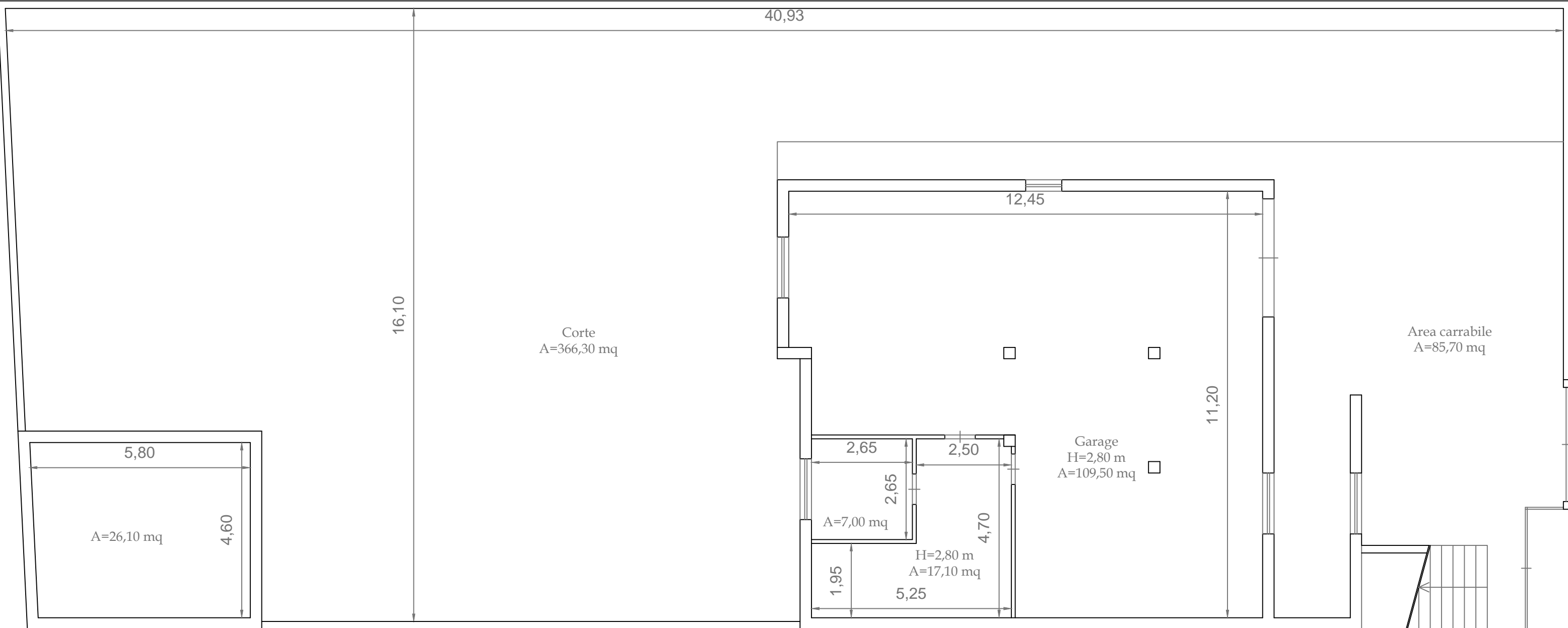
Pianta Piano Terra - Scala 1:100
