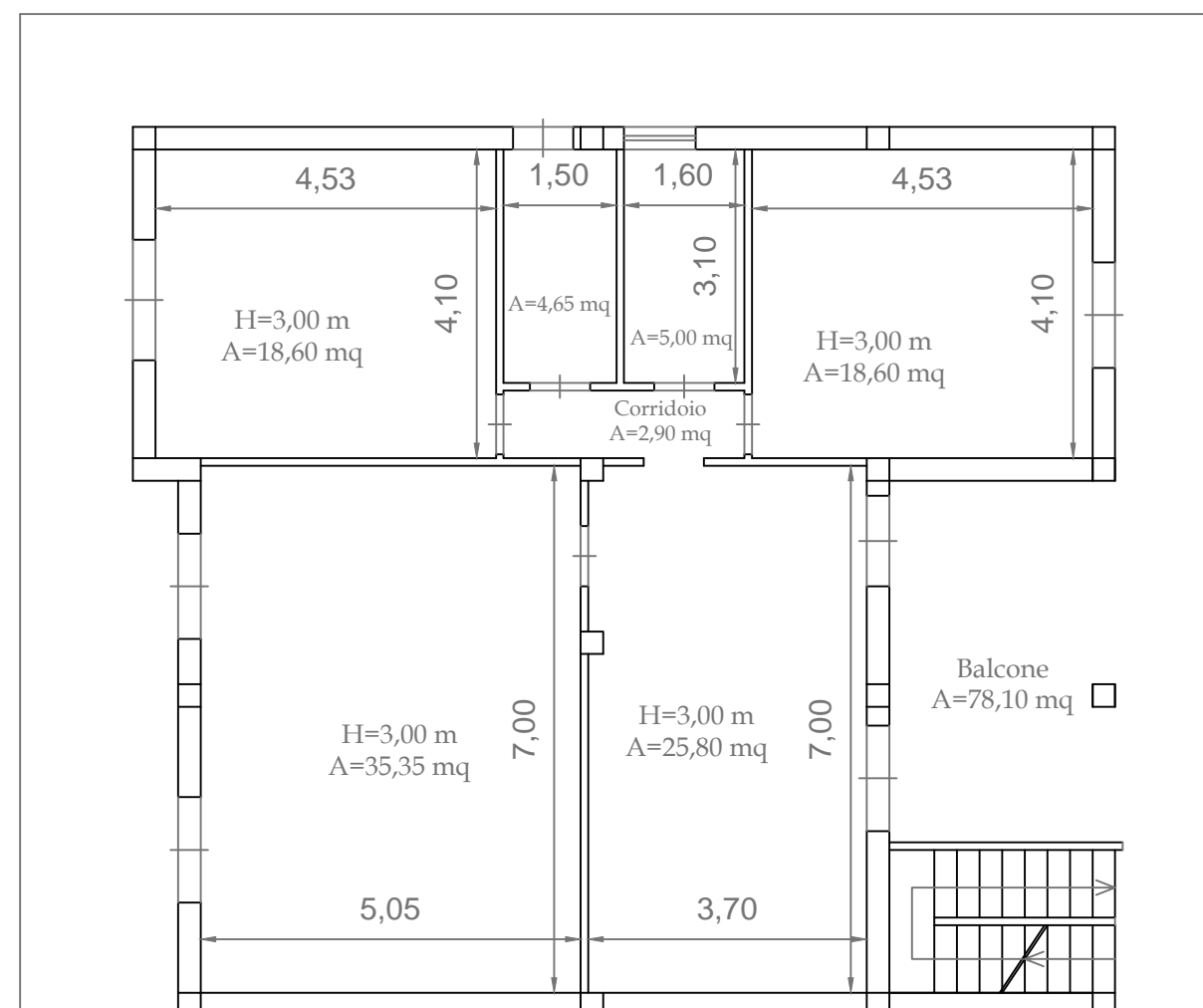
Pianta Piano Terzo - Scala 1:100
