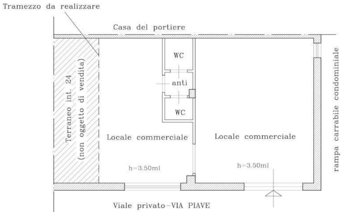
Immagine n. 3 – Pianta
