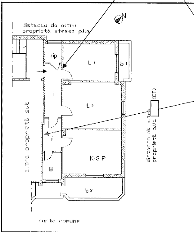
Planimetria dello stato di fatto
