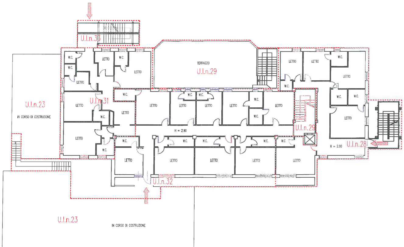
Pianta Piano Primo - 1:150
