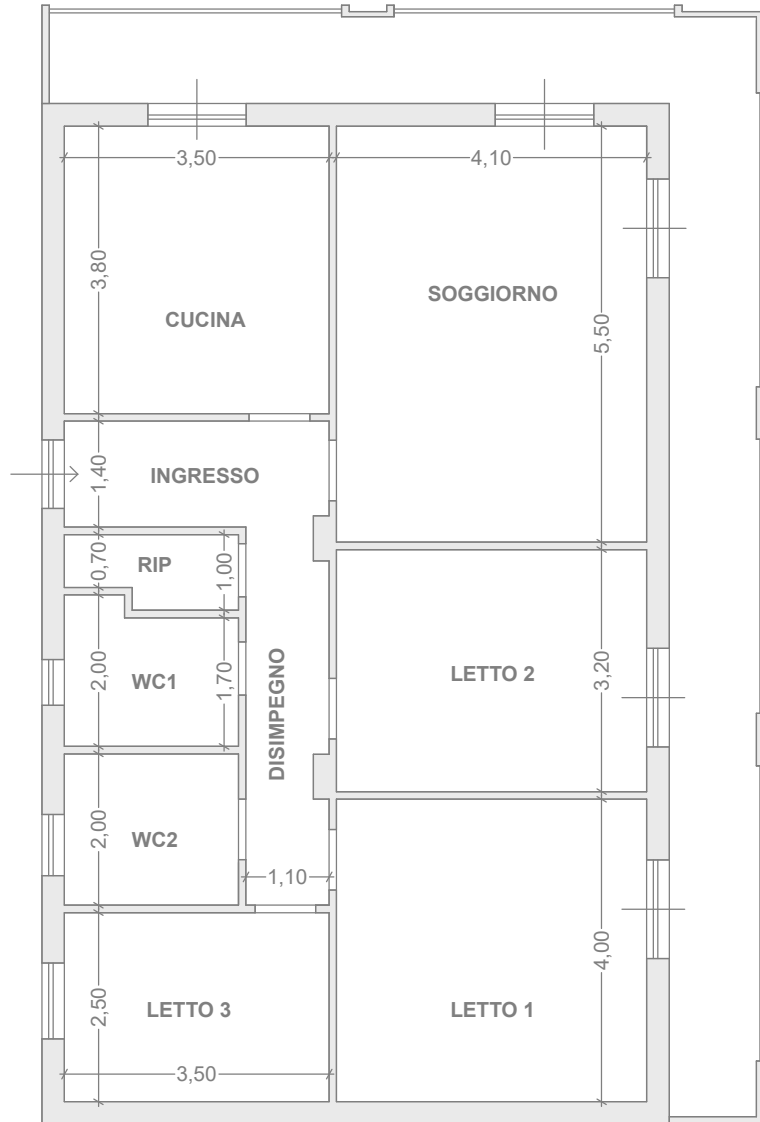
LOTTO 1 - SUB 15 - IV PIANO - RIZZA_ scala 1:100
