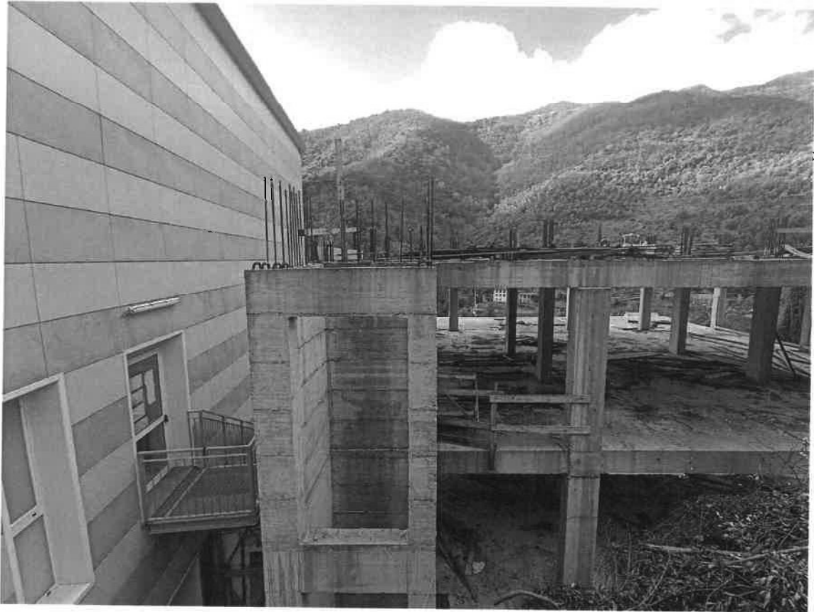
FOTO 27: BENE 2 – FABBRICATO IN COSTRUZIONE
