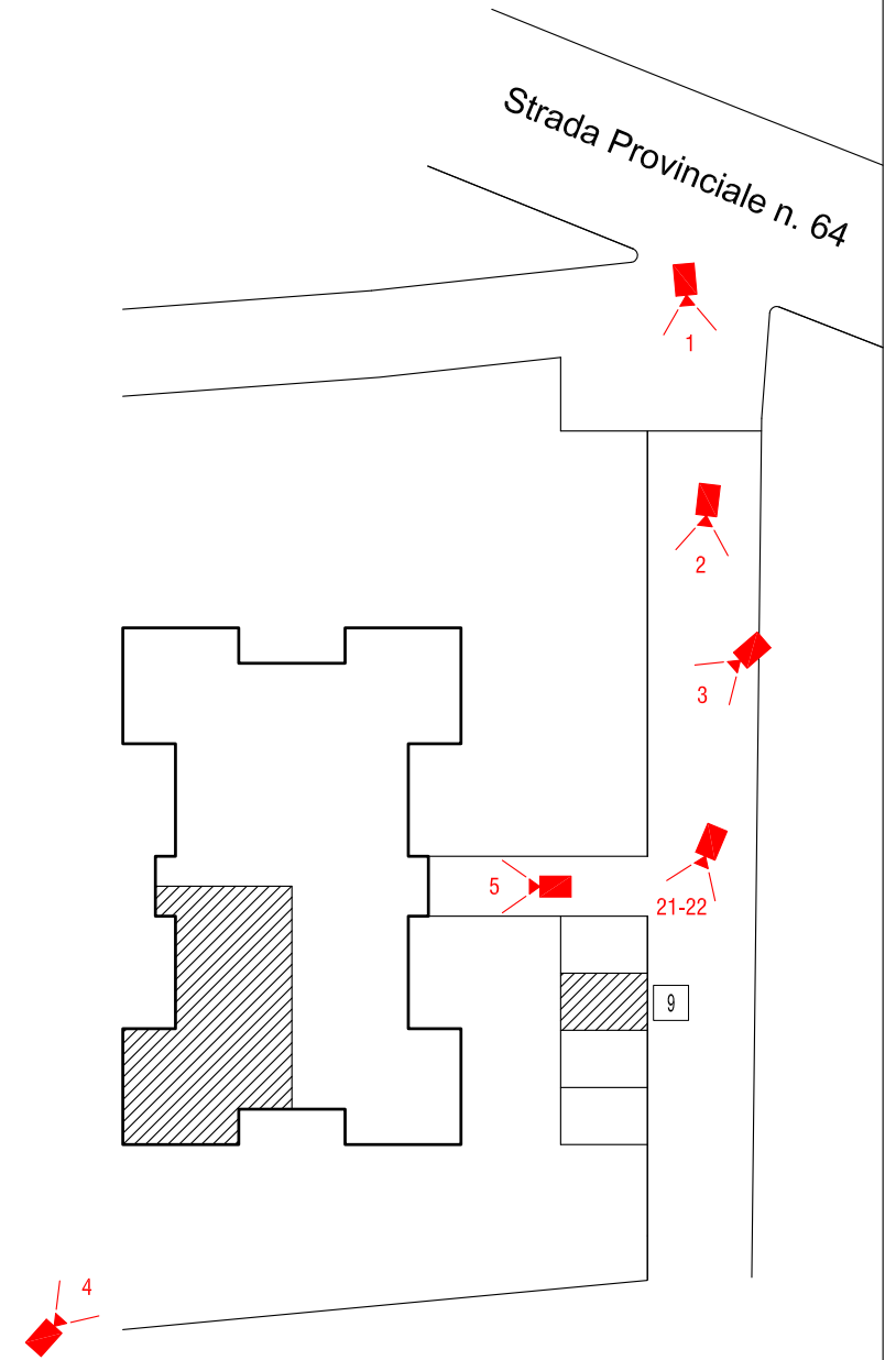
Planimetria generale 1:500
