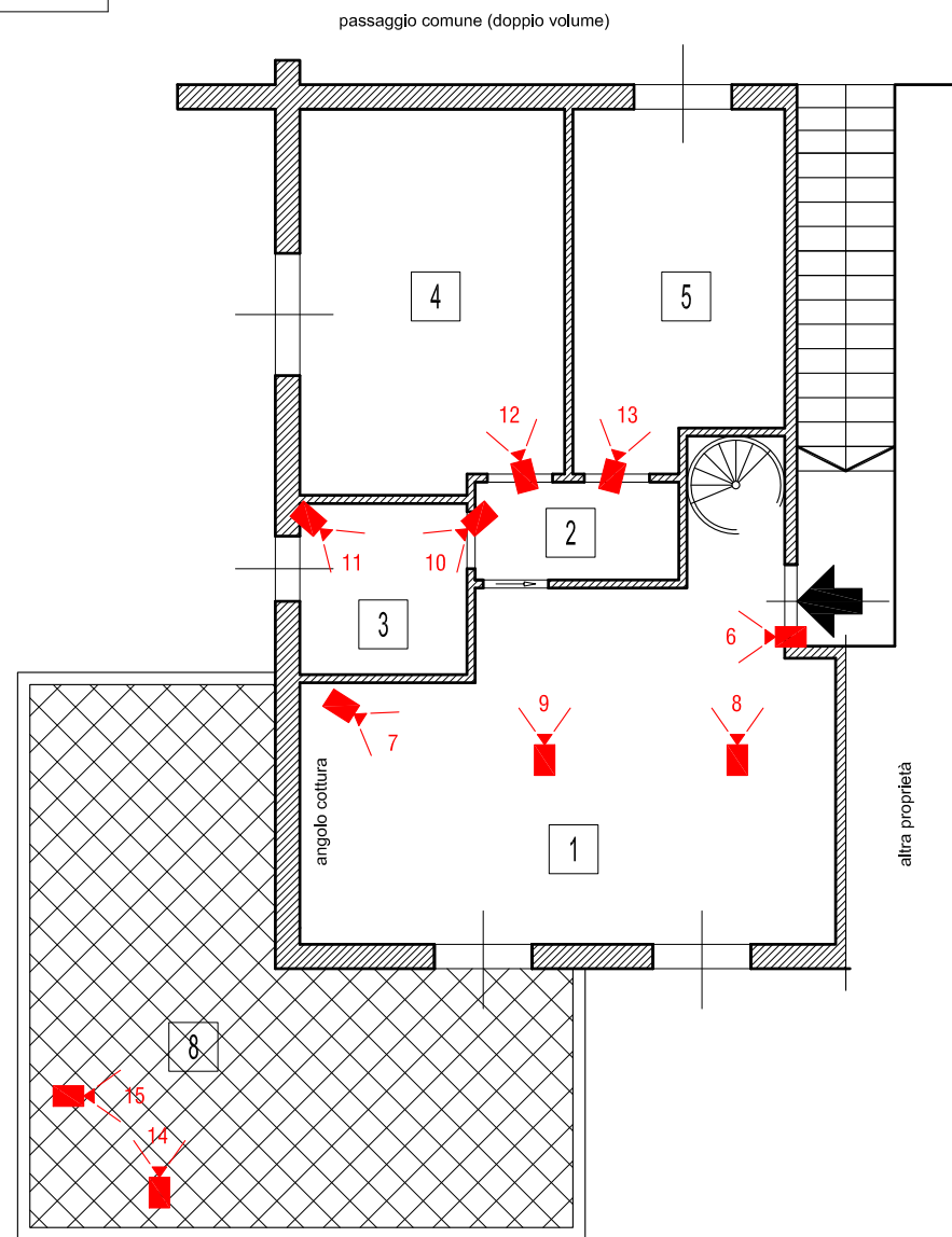
PIANO PRIMO
