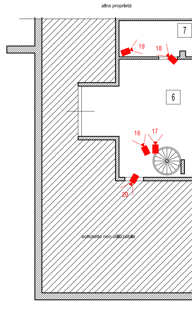
PIANO SOTTOTETTO
