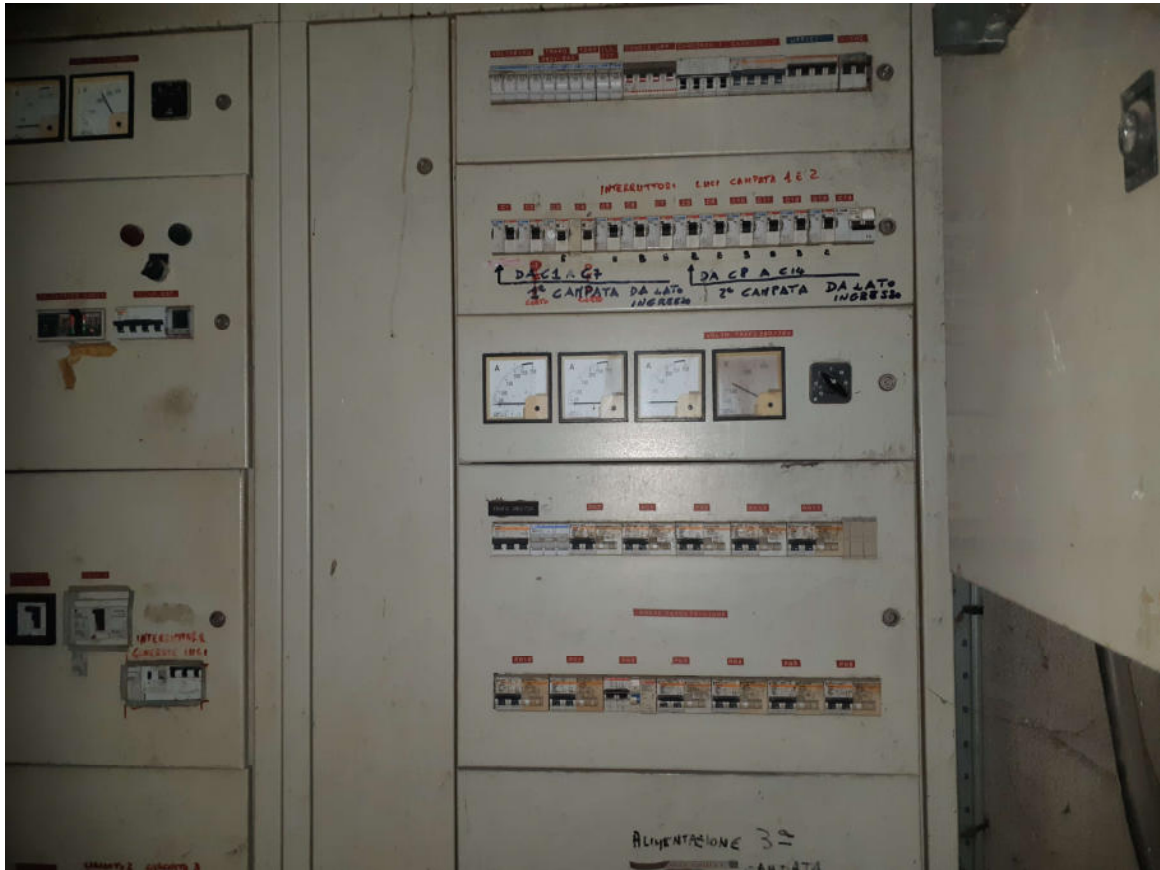
Figura 24: Quadro Elettrico all'interno del Capannone
