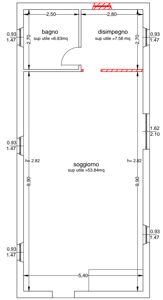
PIANO TERRA (Subalerno 4)
