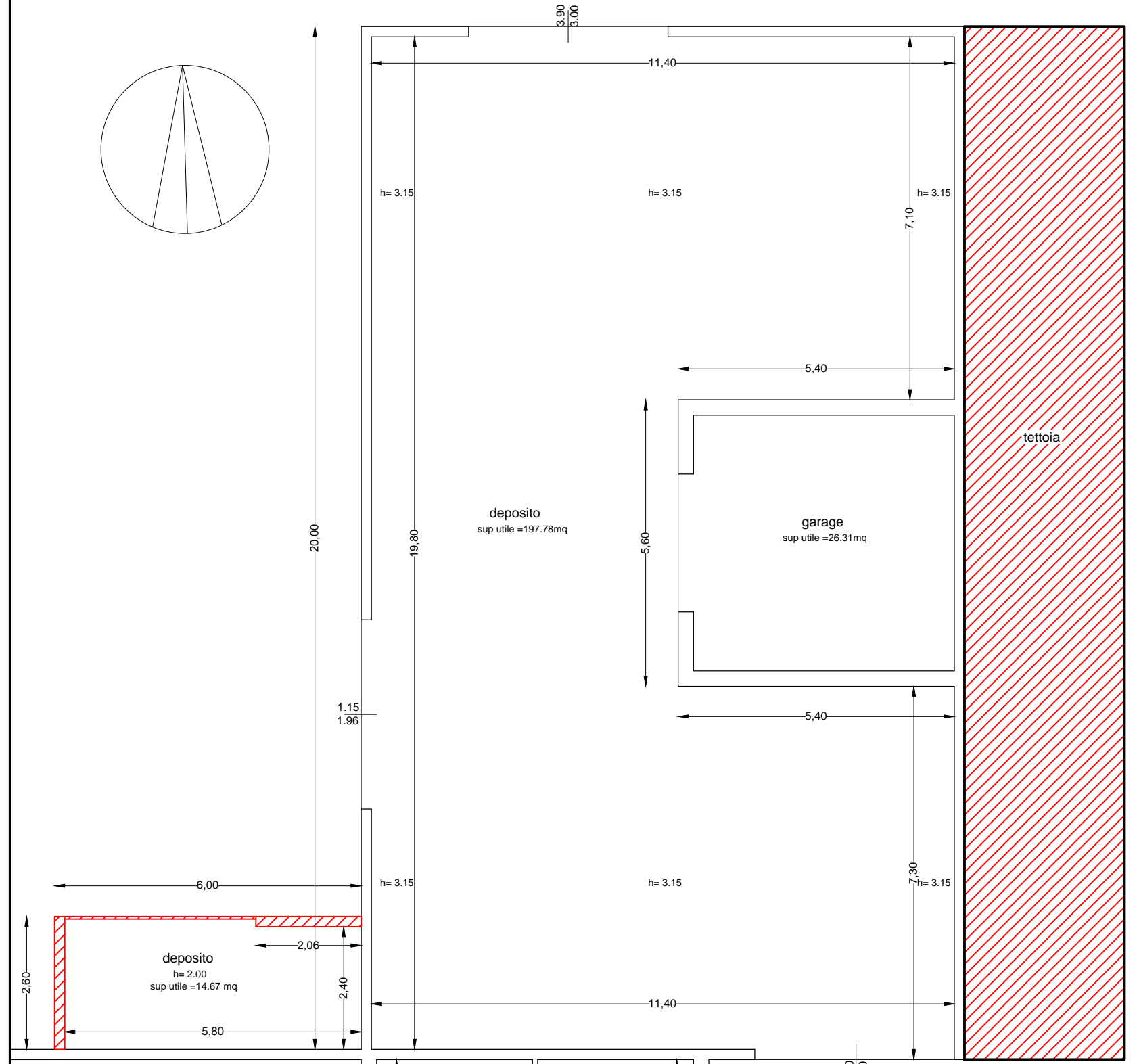
PIANO TERRA (Subalerno 5)
