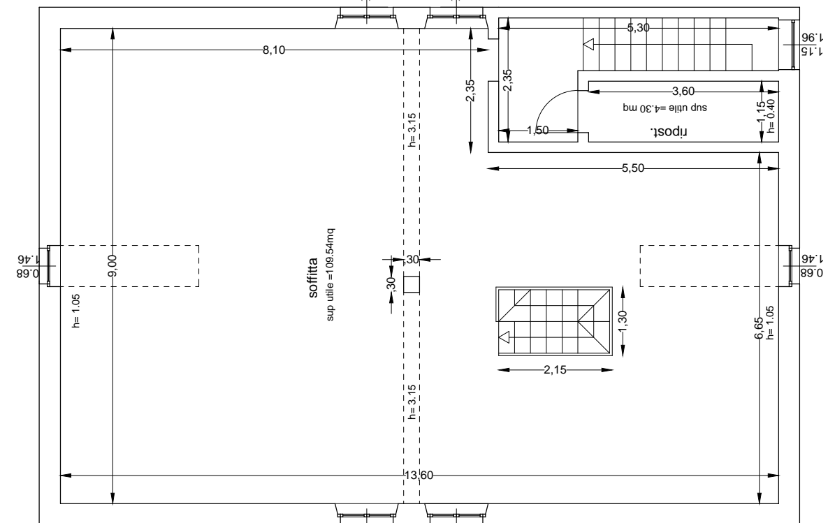
PIANO SOTTOTETTO (Subalterno n. 3)
