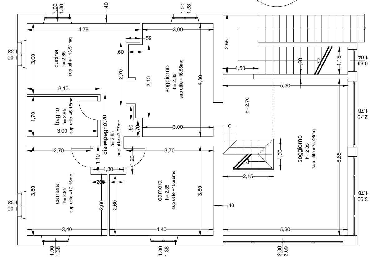
PIANO PRIMO (Subalterno n. 3)
