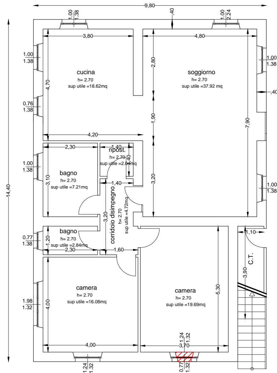
PIANO TERRA (Subalterno n. 2)
