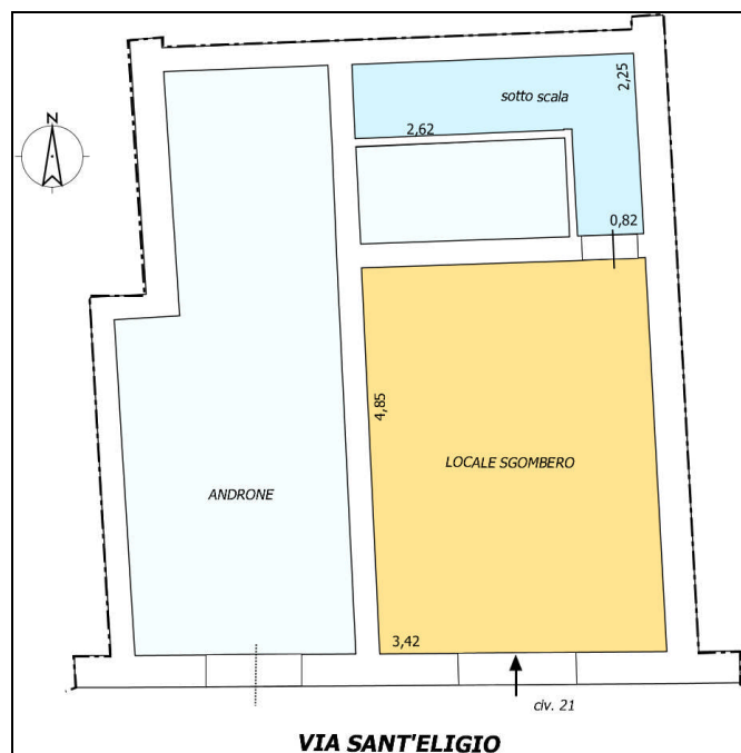
FIGURA 5 ELABORATO PLANIMETRICO LOCALE TERRANO
