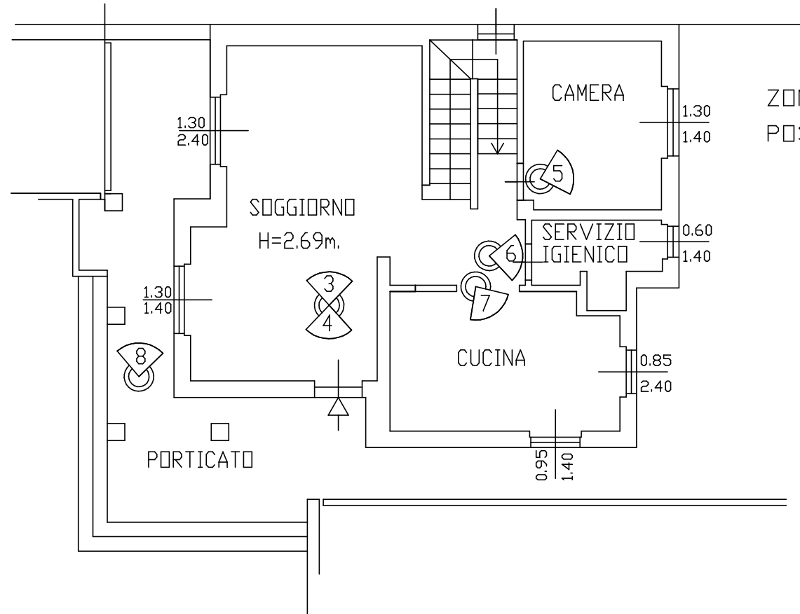
PIANO RIALZATO
