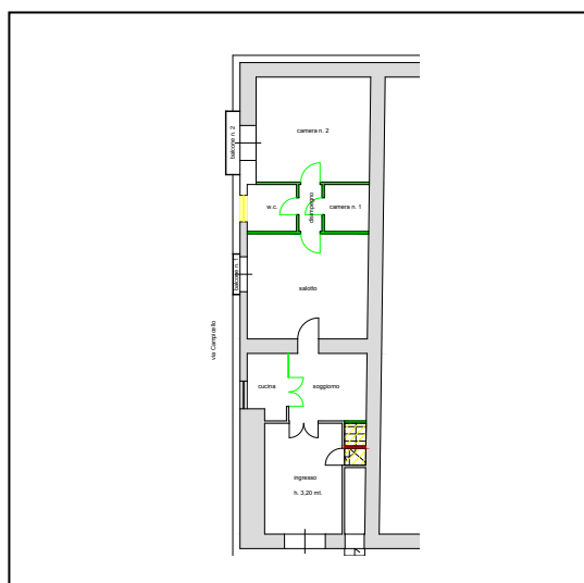
Planimetria di rilievo attuale dei luoghi con l'indicazione grafica delle difformità edilizio-urbanistiche rispetto alle planimetrie catastali d'impianto (All.13)
