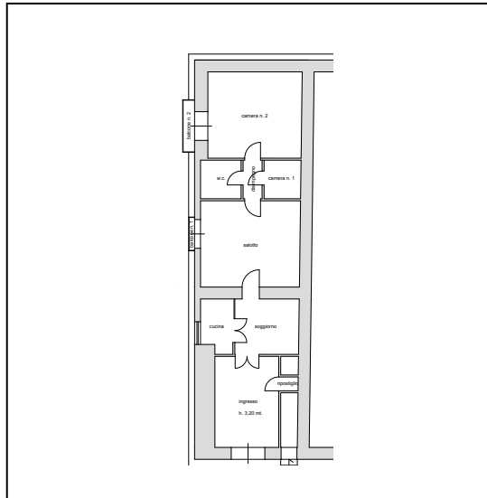
Planimetria di ripristino dello stato dei luoghi (All.14)
