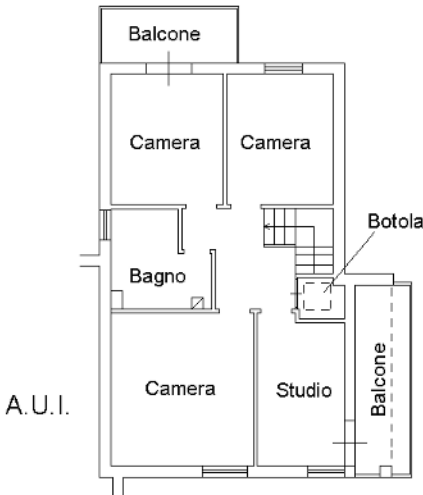
PIANTA PIANO SECONDO h 2,70 mt.
