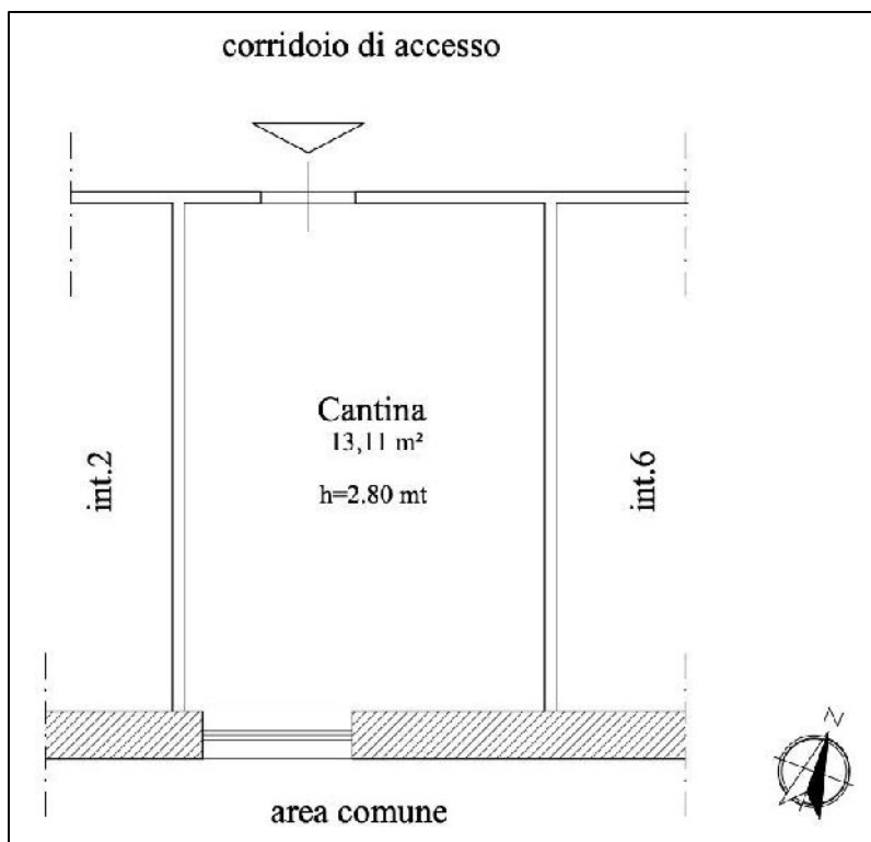
Figura 4 – Grafico dello stato dei luoghi – Cantina
