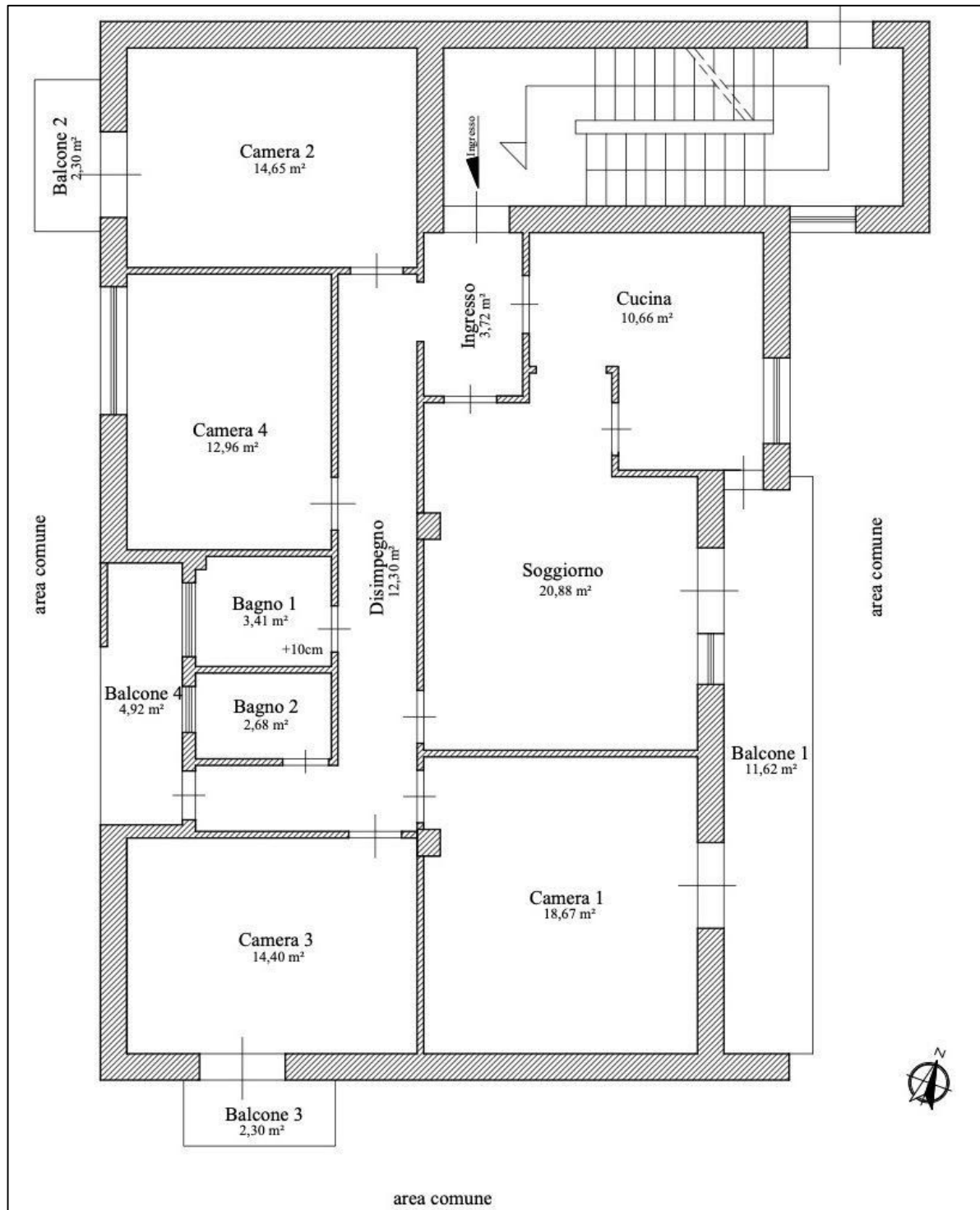
Figura 3 – Grafico dello stato dei luoghi – Appartamento - foglio 4 – p.lla 441 – Sub.5
