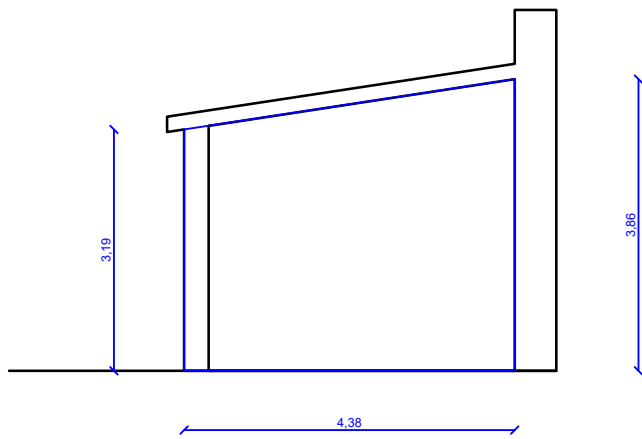
Sezione A-A scala 1:100
