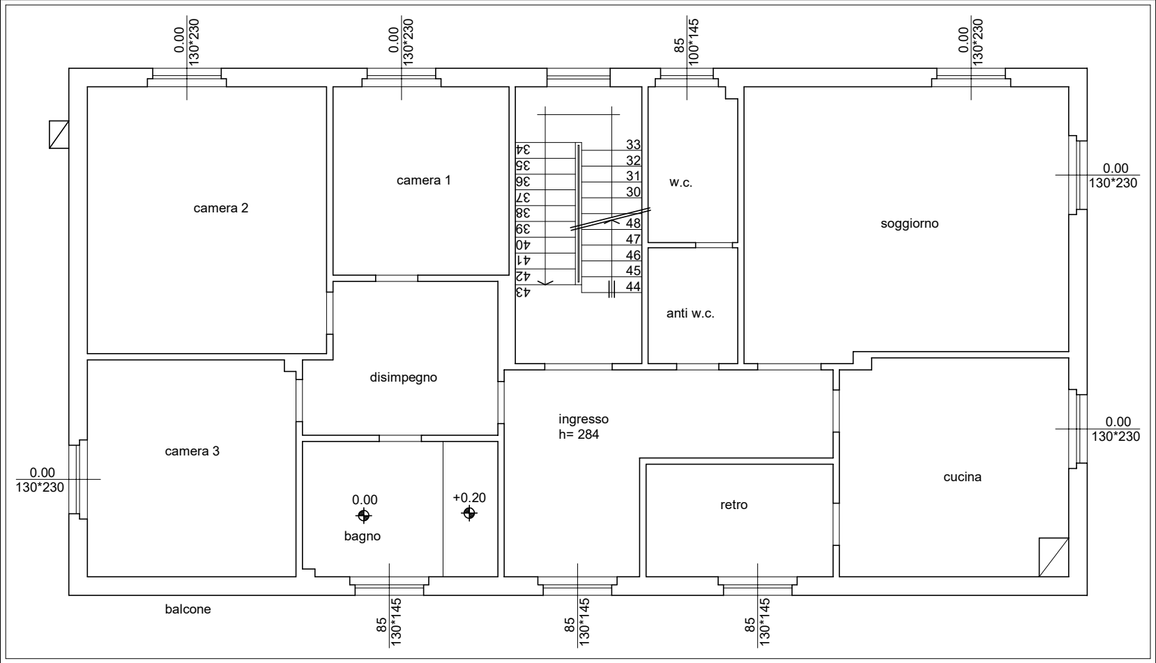
PIANTA PIANO SECONDO RAPP. 1:100
