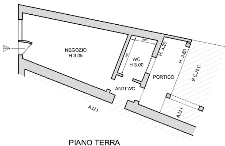
Figura 3.a Planimetria immobili sub. 3 (rilievo).
