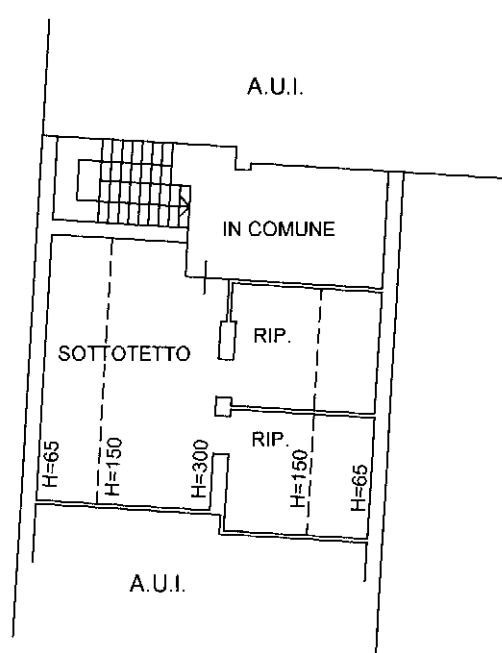
PIANO SECONDO
