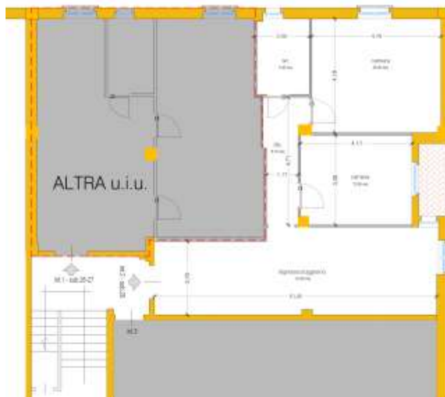
Figura 2: rappresentazione planimetria dello stato dei luoghi riscontrata in sede di sopralluogo
