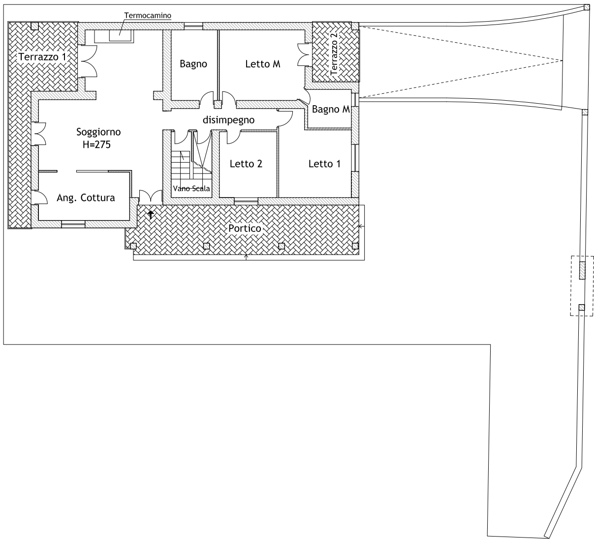
PIANO TERRA / RIALZATO - 1/200
