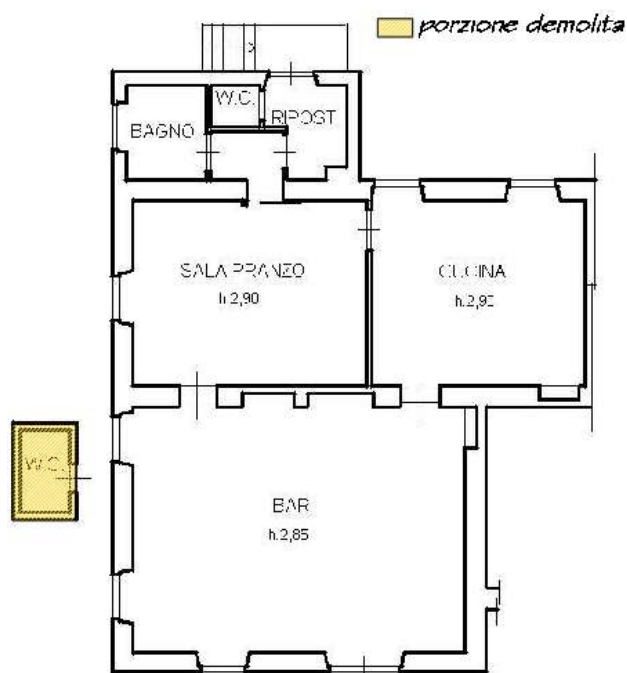
Planimetria catastale attuale
