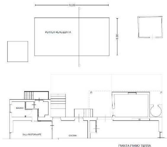
Tavola Stato finale CILA n. 502
