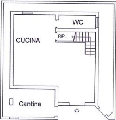
PIANO INTERRATO H. 2,70
