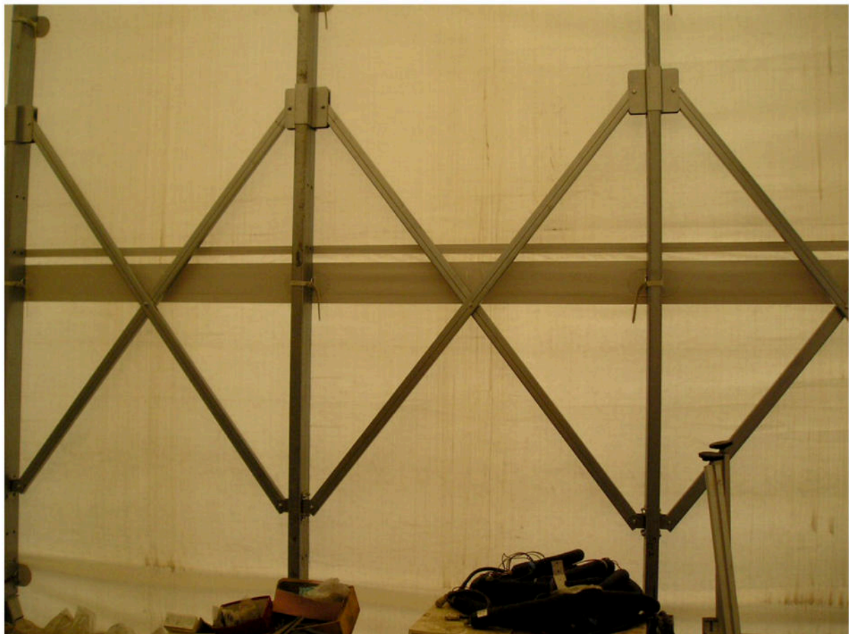
Fotografia 32 - Interno Struttura Telonata
