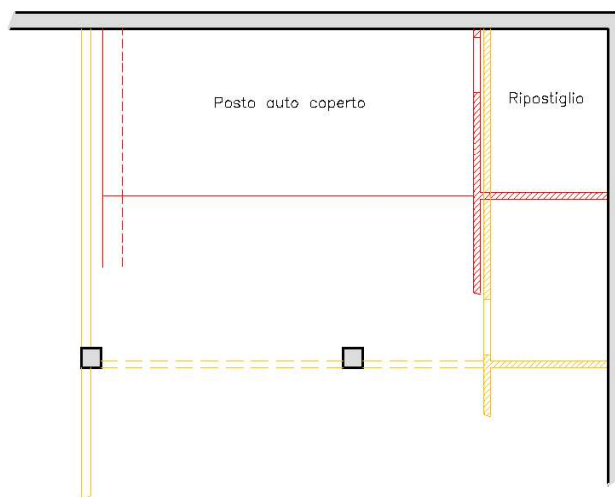
PIANO SEMINTERRATO – Stato Sovrapposto
