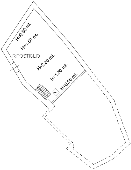
PIANO QUARTO (SOTTOTETTO)
