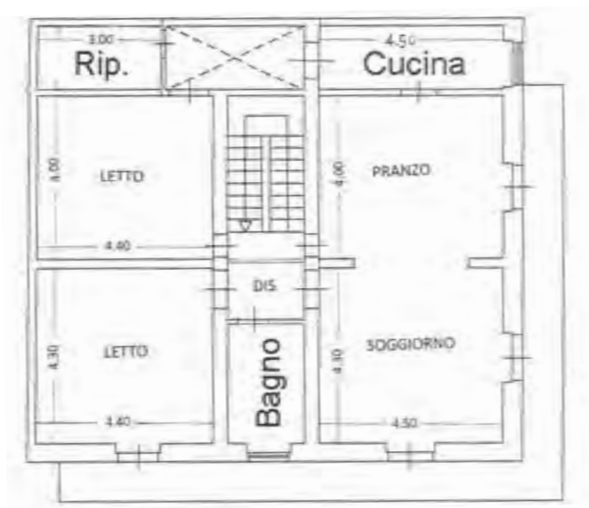
Rilievo dello stato di fatto - Pianta piano primo
