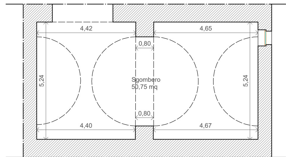
Pianta piano interrato
