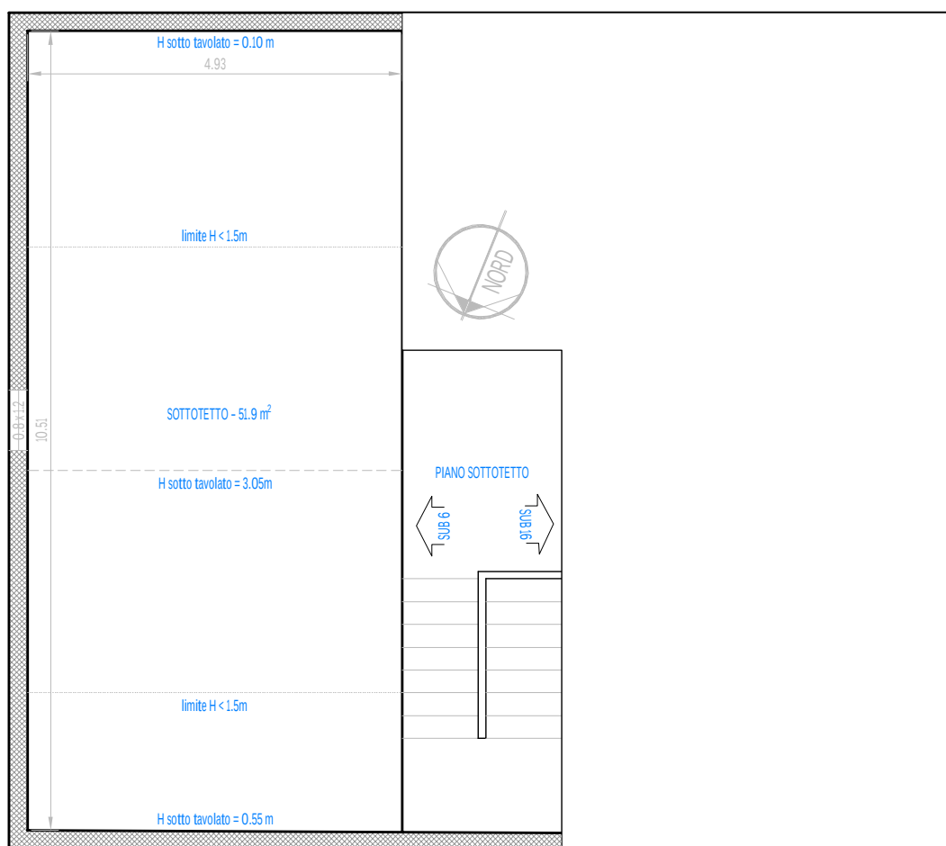
Planimetria di rilievo dello stato di fatto – Sottotetto
