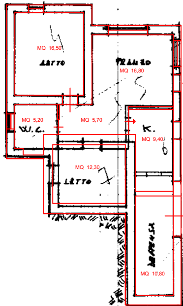
PIANTA PIANO SOTTOSTRADA PRIMO h=m. 2.85
