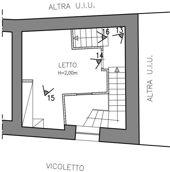
Piano Ammezzato
