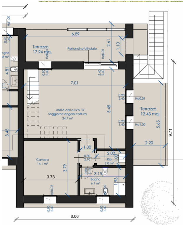
piano primo
