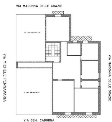
PIANO SECONDO
