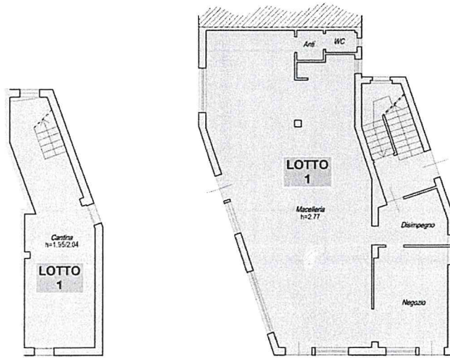
PIANTA PIANO SOTTOSTRADA
