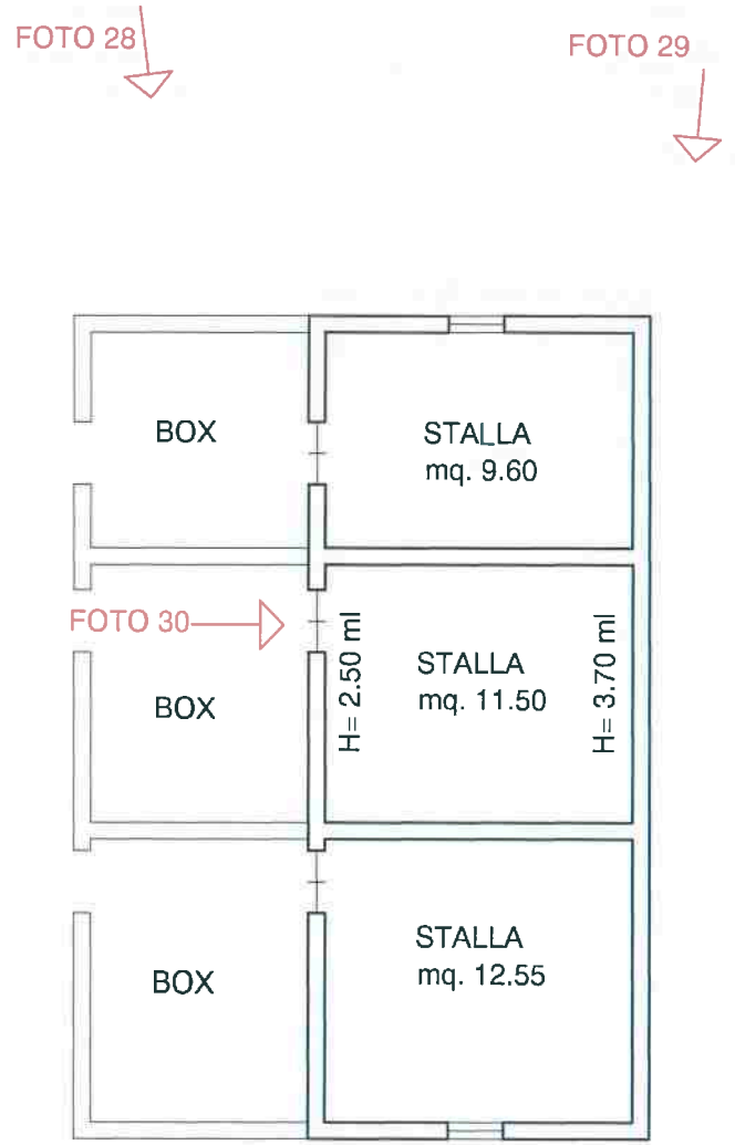
PIANTA PIANO TERRA FABBRICATO ACCESSORIO A
