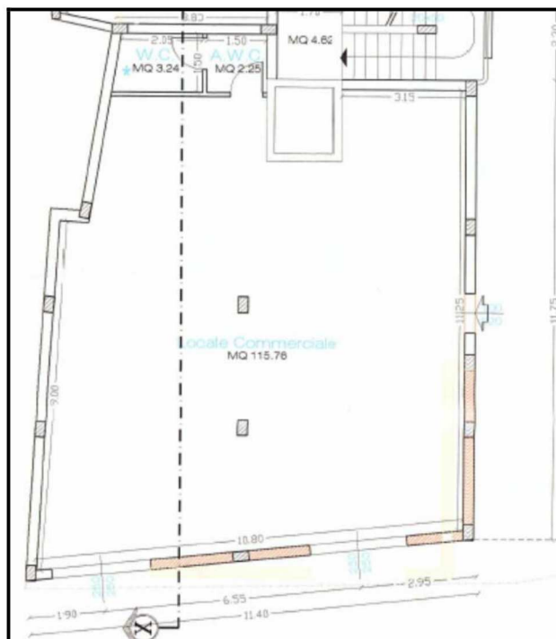
Pianta del piano terra (progetto)
