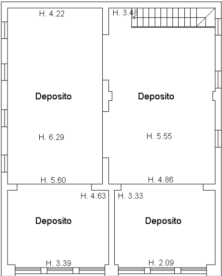
PIANO PRIMO
