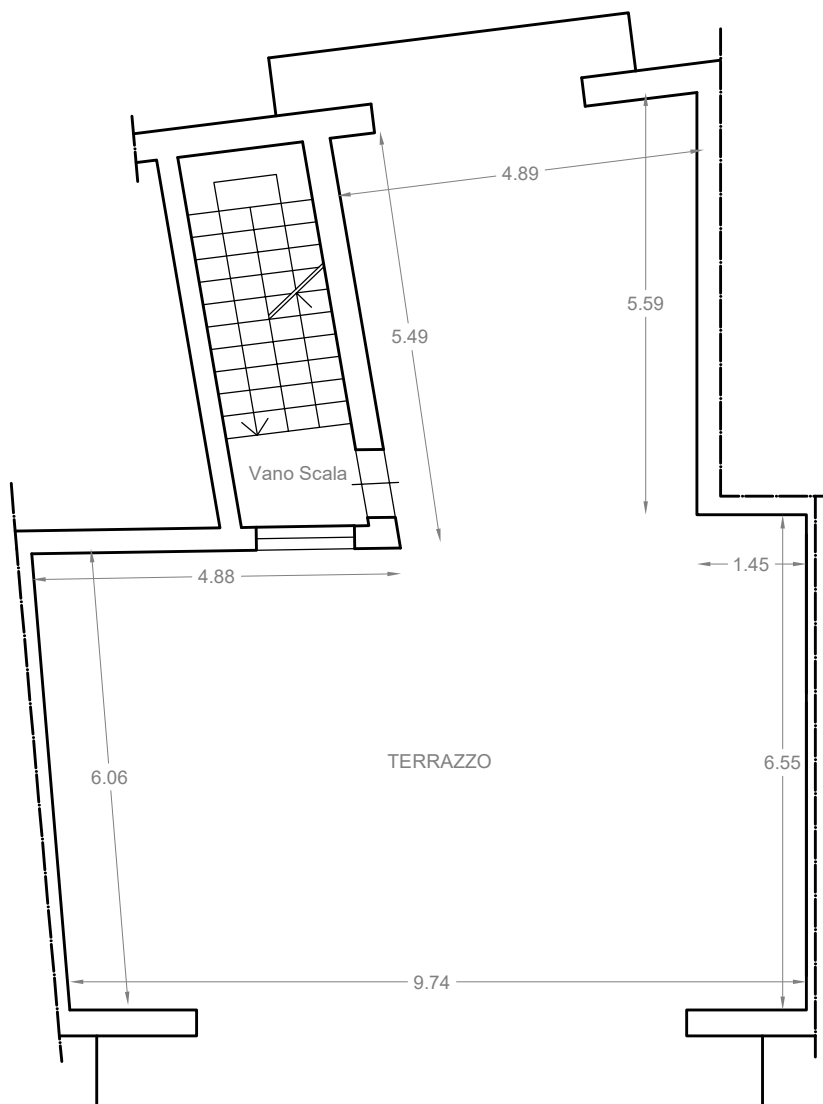
PIANTA PIANO COPERTURA SC. 1:100
