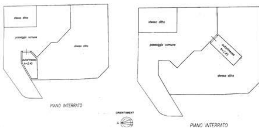
estratto planimetria sub 7
