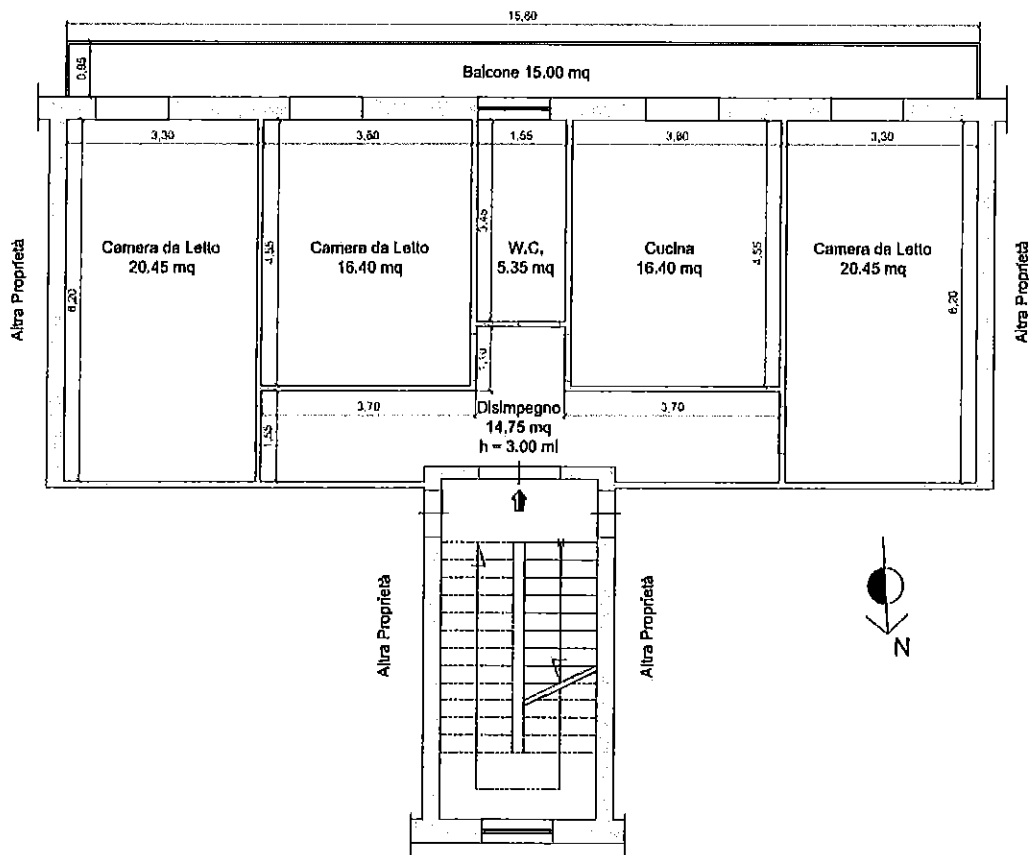
Figura 3 - Planimetria Catastale Abitazione Piano Primo.
