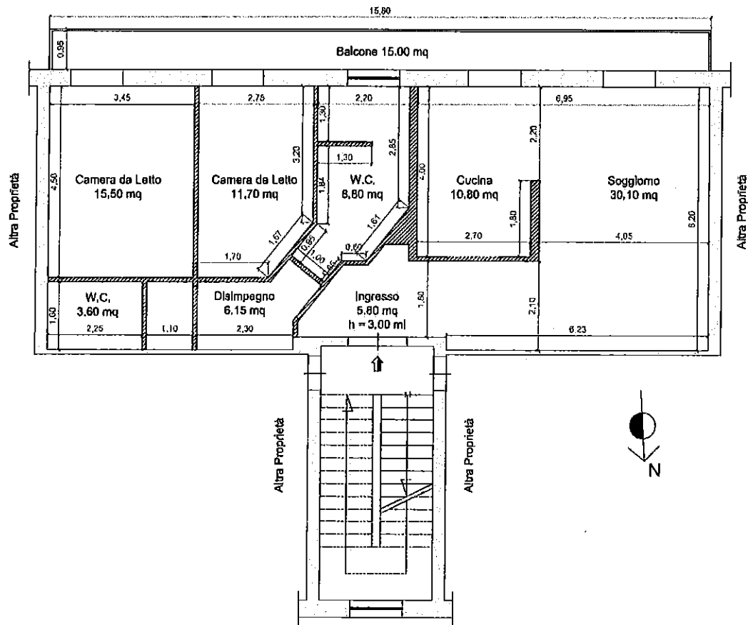
Figura 5 - Planimetria Stato di Fatto Abitazione Piano Primo.
