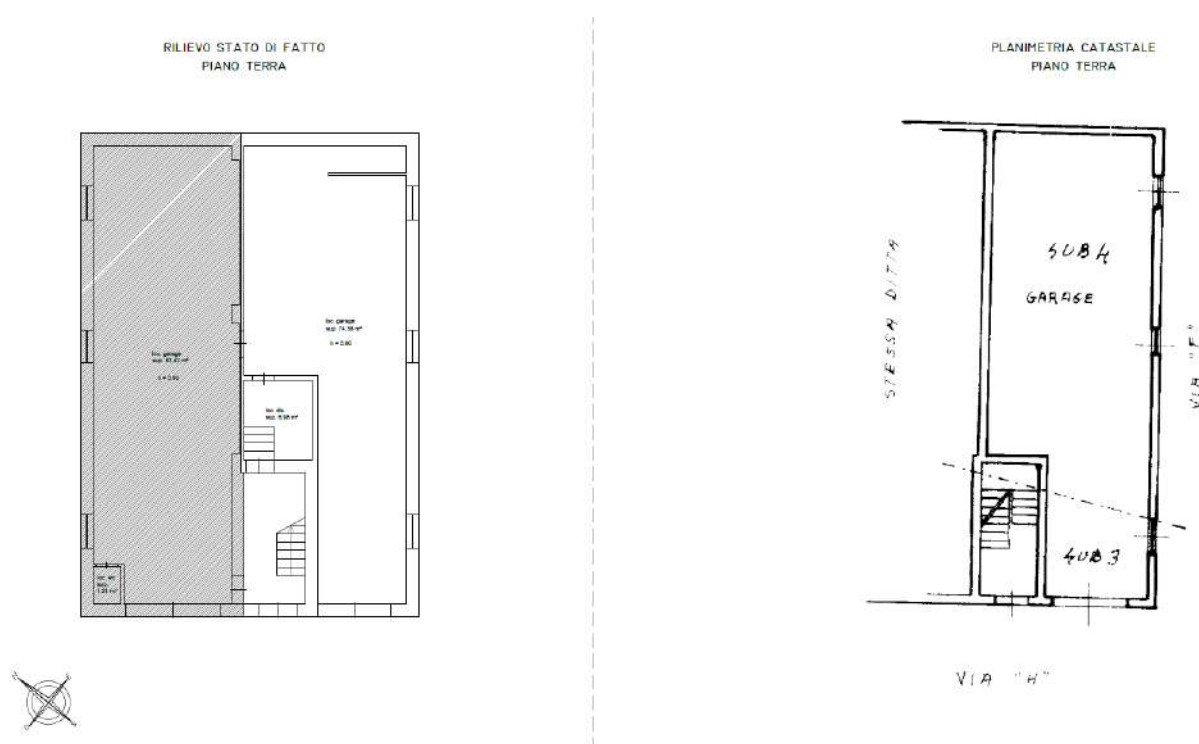
Figura 7 - Confronto rilievo stato di fatto con pln catastale (tav. H)
