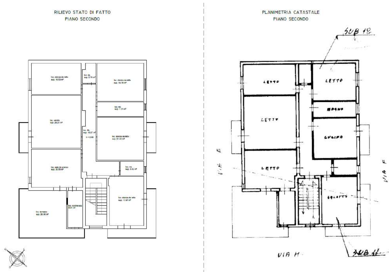
Figura 13 – Confronto rilievo stato di fatto con pln catastale (tav. M)
