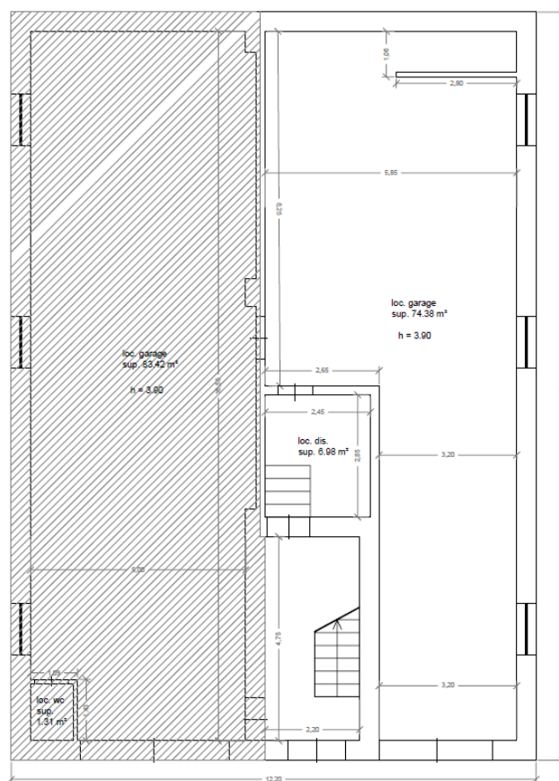
Figura 16 – Rilievo stato dei luoghi (Tav. B)
