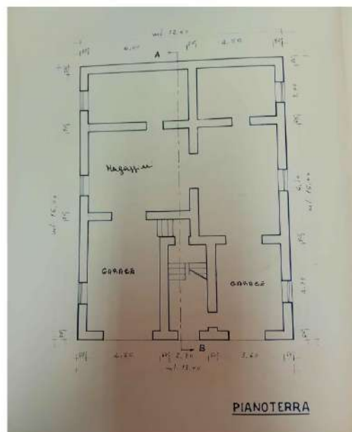
Figura 20 – Confronto rilievo stato dei luoghi con planimetria urbanistica _ Piano Terra (Tav. N)
