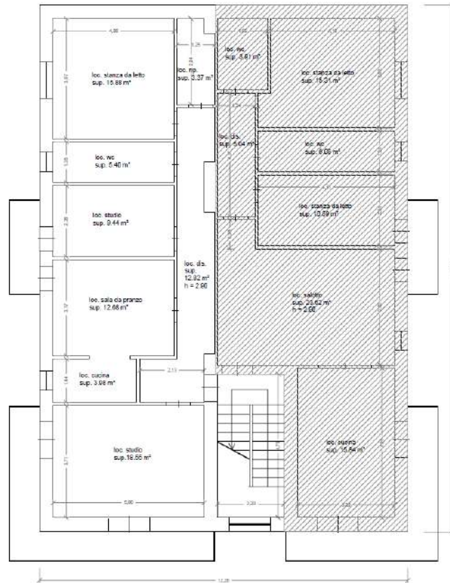
Figura 17 – Rilievo stato dei luoghi (Tav. C)
