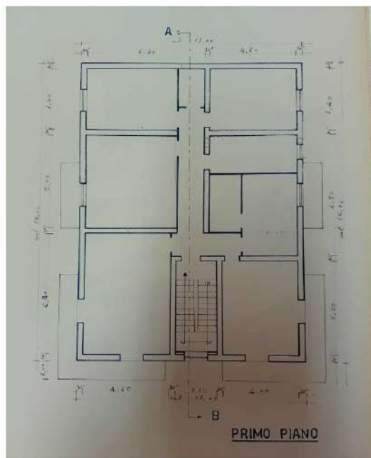
Figura 21 – Confronto rilievo stato dei luoghi con planimetria urbanistica _ Piano Primo (Tav. O)
