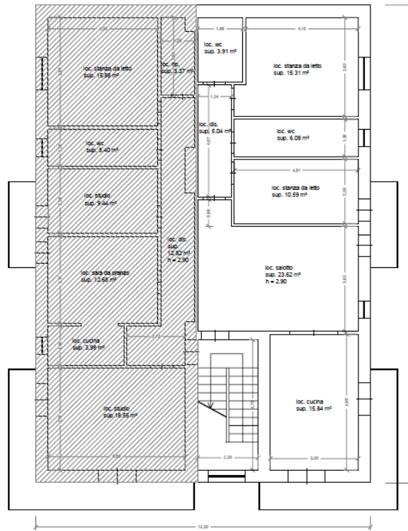
Figura 18 – Rilievo stato dei luoghi (Tav. D)
