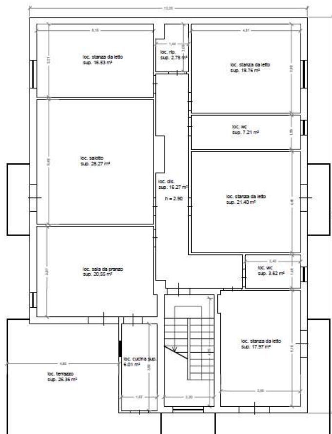
Figura 19 – Rilievo stato dei luoghi (Tav. E)
