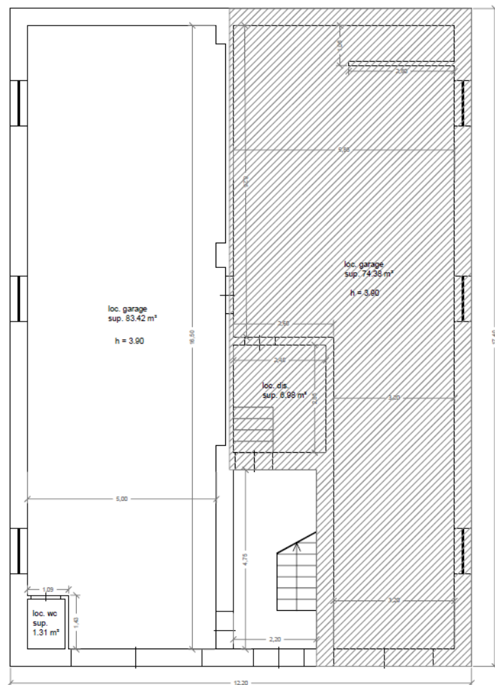
Figura 15 – Rilievo stato dei luoghi (Tav. A)
