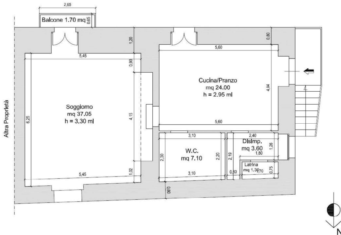
Figura 3 - Planimetria Catastale Piano Terra, Foglio 20, p.lla 161, Sub 4.
