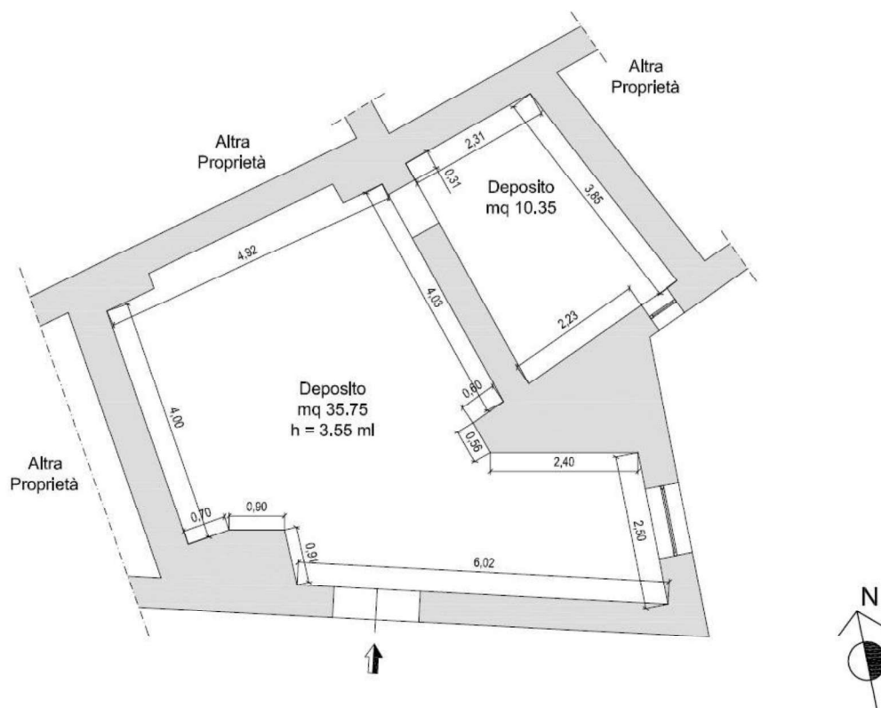
Figura 4 - Planimetria Catastale Piano Terra, Foglio 20, p.lla 124, Sub 14 (Graffata con p.lla 130, sub 5).
