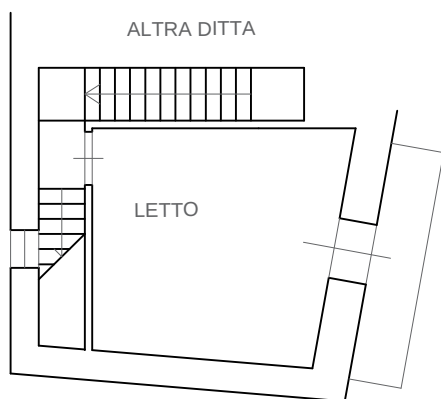
PIANTA PIANO PRIMO H=2.40
