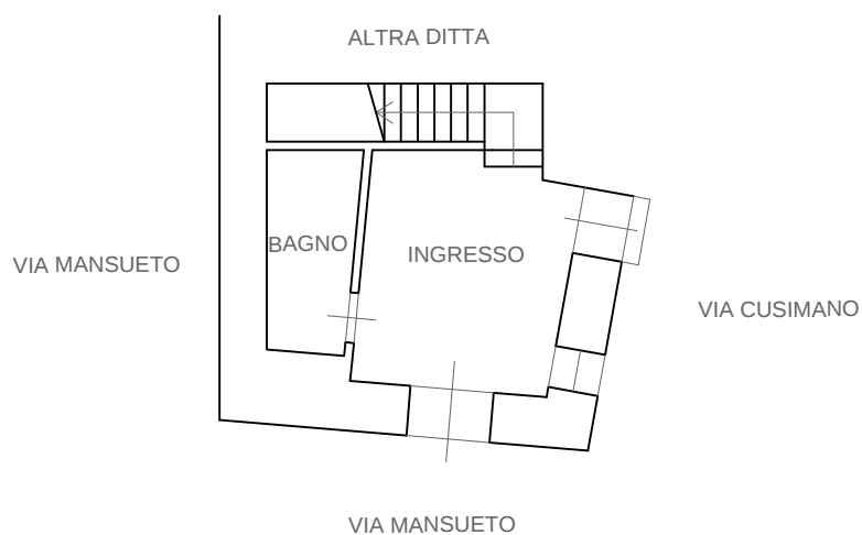
PIANTA PIANO TERRA H=2.55
