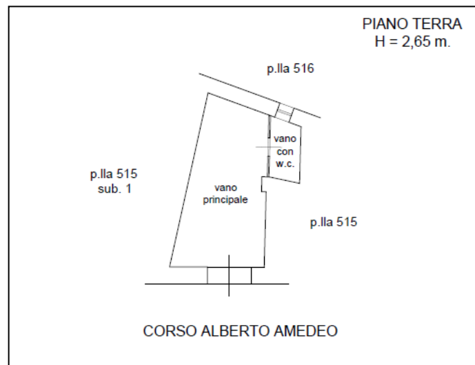
Planimetria di rilievo dello stato di fatto (All. 7) – Scala 1:200
