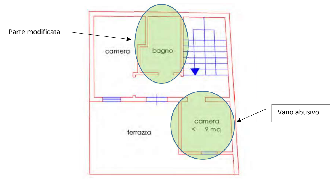
PIANTA PIANO SECONDO STATO DI FATTO
