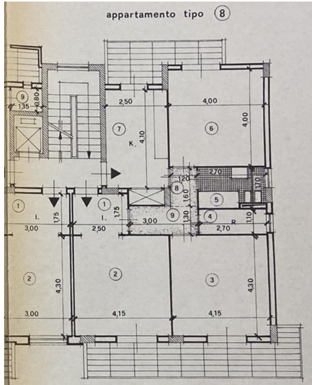
Stralcio della planimetria di progetto originario approvato dalla C.E. il 14/01/1977
