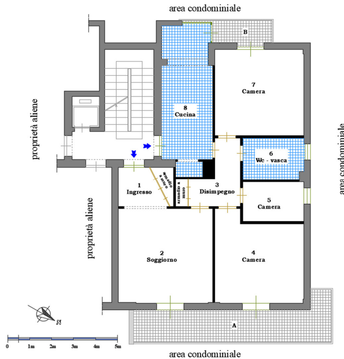
Planimetria di rilievo dello stato di fatto
