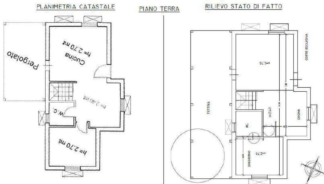
FIGURA 14 - CONFRONTO PLANIMETRIA CATASTALE CON STATO DI FATTO PT
