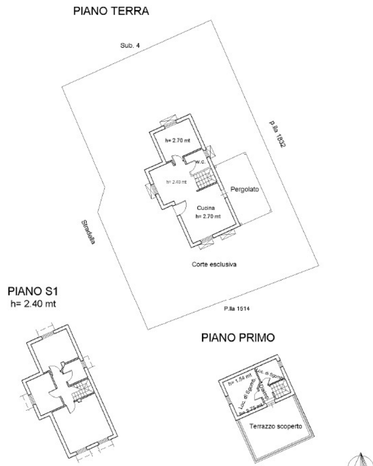
FIGURA 13 – PLANIMETRIA CATASTALE
