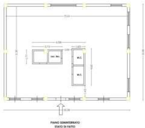
Stato di fatto – Piano Seminterrato
