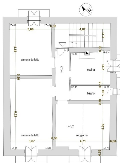
Pianta di rilievo
